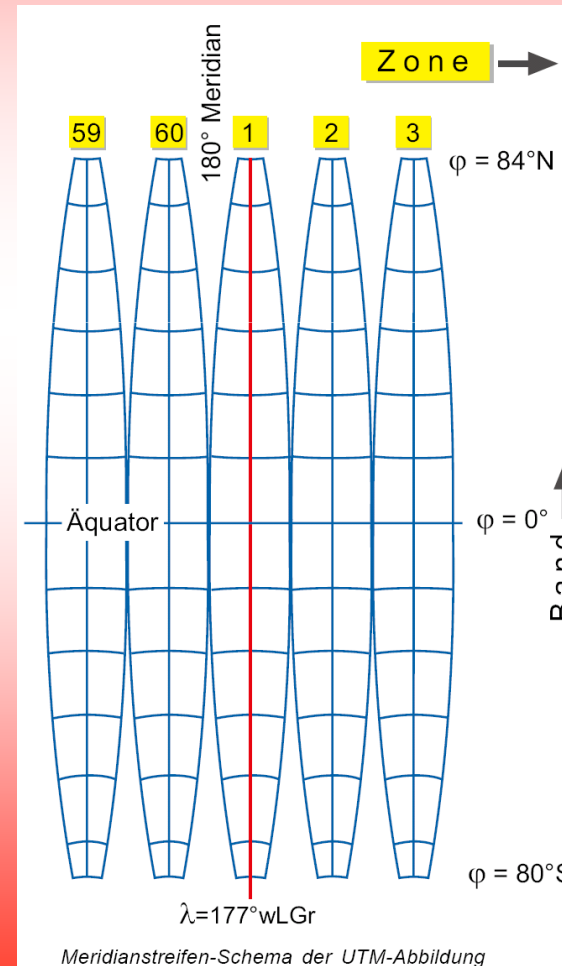
Meridianstreifen-Schema der UTM-Abbildung
